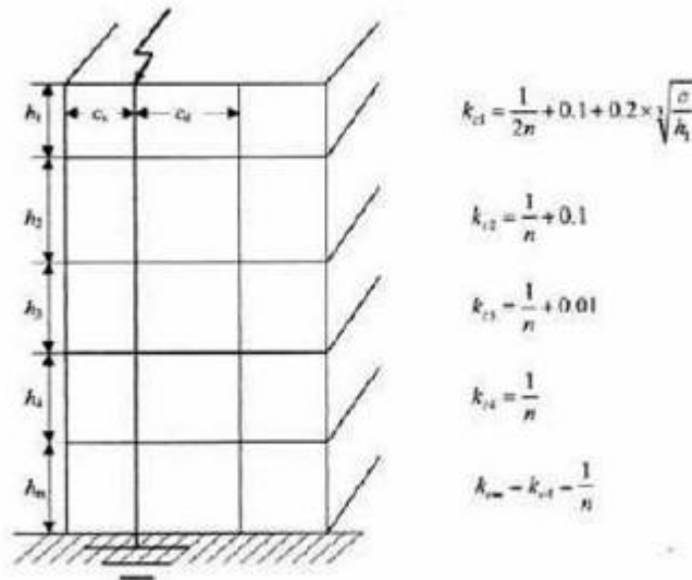
图 E.0.2 分流系数 k_c (2)
