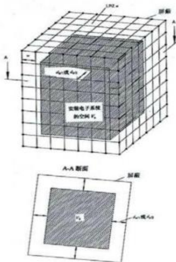
图 6.3.2-2 在 LPZn 区内供安放电气和电子系统的空间 注: 空间 V_s 为安全空间
