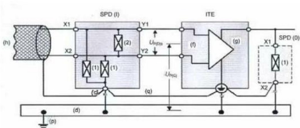
图 J. 2. 3-1 防需要保护的电子设备 (ITE) 的供电电压输入端
