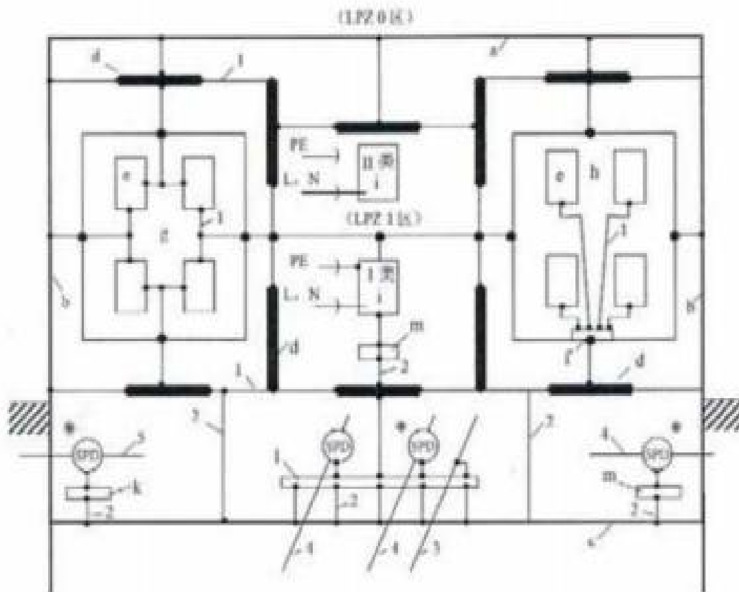
图 6.3.3 接地、等电位连接和接地系统的构成
