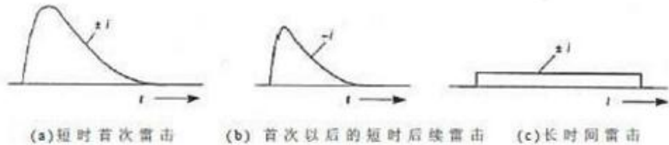
F.0.1-1 闪电中可能出现的三种雷击
