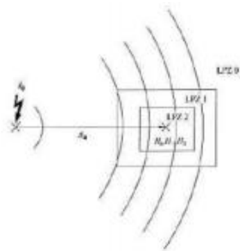
图 6.3.2-1 附近雷击时的环境情况
